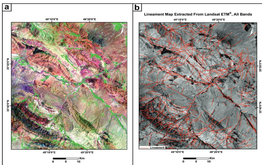
شکل ۳. الف) تصویر رنگی نسبت بانندی 321=RGB منطقه مورد مطالعه با ماهواره لندست، ب) خطواره‌های استخراج شده از تصاویر لندست
