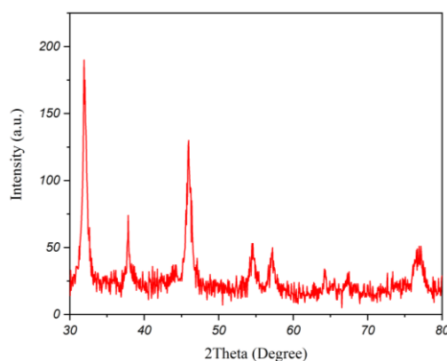
شکل ۲- الگوی XRD نانوذرات سنتز شده با روش اولتراسونیک. دمای ۲۵ درجه سانتی گراد و pH اسیدی ۴
