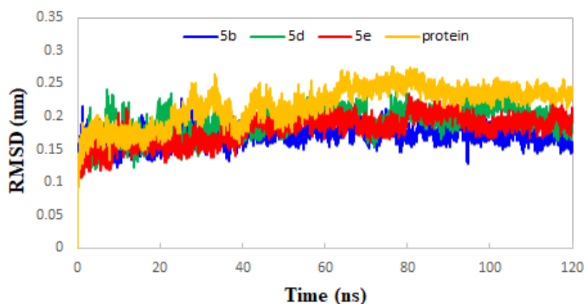
شکل ۲- RMSD کربن های آلفا COX-2 در سیستم های شبیه سازی شده.
