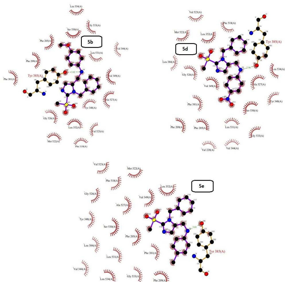
شکل ۱- نمودار LIGPLOT لیگاند های 5b، 5d و 5e؛ برهمکنش های پیوند هیدروژنی بین پروتئین و لیگاند با خط چین (سبز) و برهم کنش های هیدروفوبیک توسط کمان قرمز رنگ نمایش داده می شوند.
