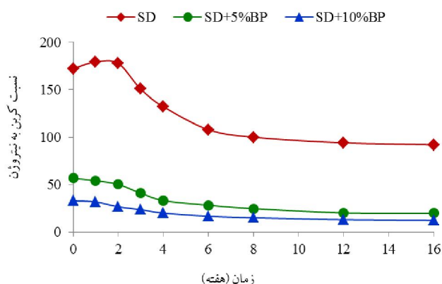
شکل ۶- روند زمانی تغییرات نسبت کربن نیتروژن خاکاره (SD) تیمار شده با سطوح مختلف پودر خون (BP) طی فرایند ورمی کمپوست سازی.
