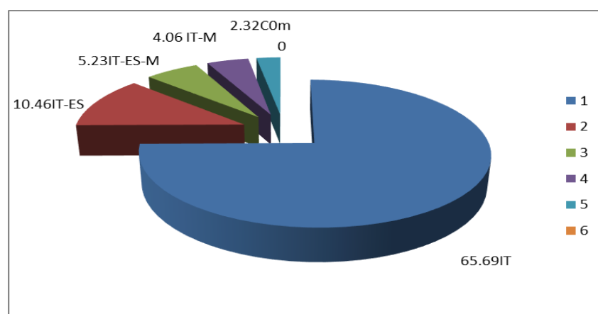
شکل ۴- نمودار درصد کوروتیپ گونه‌ها در منطقه تنگ سرخ. IT: ایرانو-تورانی، It-Es: ایرانو-تورانی/ اروپا سبیری، It-Es-M: ایرانو-تورانی/ اروپا سبیری/ مدیترانه ای، Com: همه جازی، It-M: ایرانو-تورانی/ مدیترانه ای، Cosm: کوسمپولیتان.
