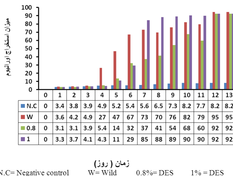
شکل ۱- میزان استخراج اورانیوم توسط باکتری وحشی در مقایسه با باکتری جهش یافته با ۱٪ (V/V) و ۰.۸٪ (V/V) DES: N.C) کنترل منفی، W: باکتری وحشی، ۰.۸٪ (V/V) جهش ناشی از ۱٪ (V/V) DES، ۰.۸٪ (V/V) جهش ناشی از ۰.۸٪ (V/V) DES.
