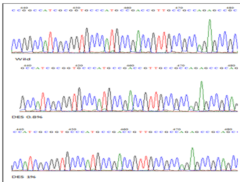
شکل ۶- گراف ترسیم شده توسط نرم افزار Bioedit توالی باکتری اسیدیتوباسیلوس فرواکسیدانس قبل و بعد از جهش با ۱٪ (V/V) و ۰.۸٪ (V/V) DES.
