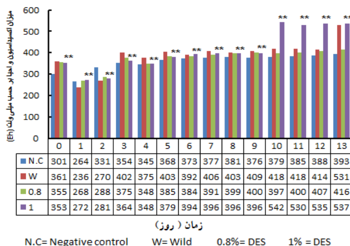
شکل ۳- میزان اکسیداسیون و احیا توسط باکتری وحشی در مقایسه با باکتری جهش یافته با ۱٪ (V/V) و ۰٫۸٪ DES. N.C: کنترل منفی، W: باکتری وحشی، ۰٫۸٪: جهش ناشی حاصل از ۰٫۸٪ DES (V/V)، ۱٪: جهش ناشی از ۱٪ DES (V/V). علامت ** نشان‌دهنده نتیجه حاصل از تحلیل آماری باکتری جهش یافته با ۱٪ DES بوده که با باکتری وحشی معنی‌دار هستند ( P < 0.05 ).
