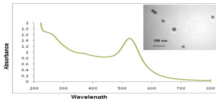
شکل ۲- طیف UV-Vis و تصویر TEM نانوذرات ۱۰ نانومتر به کار رفته در مطالعه اخیر.
