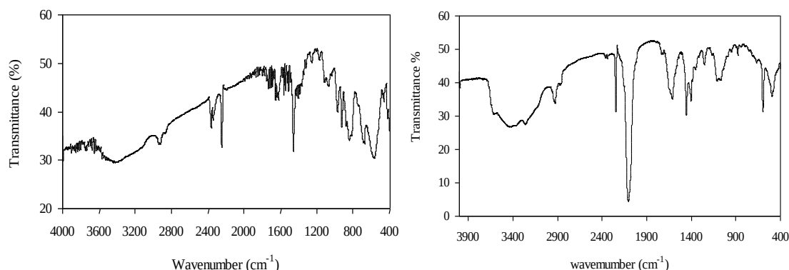
شکل ۱. طیف IR (سمت راست) برای کامپوزیت سریم مولیبدات-پلی اکریلونیتریل و (سمت چپ) برای کامپوزیت مس هگزاسیانوفرات-II- پلی اکریلونیتریل
