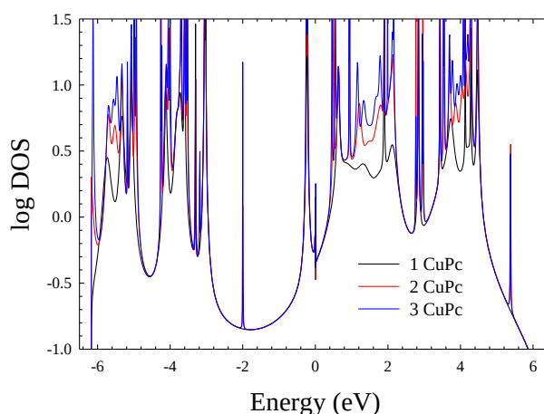
شکل ۴. (آنلاین رنگی) لگاریتم چگالی حالت‌های الکترونی سامانه‌های شامل یک، دو و سه مولکول فتالوسیانین مس متصل شده به دو هادی فلزی، بر حسب انرژی
