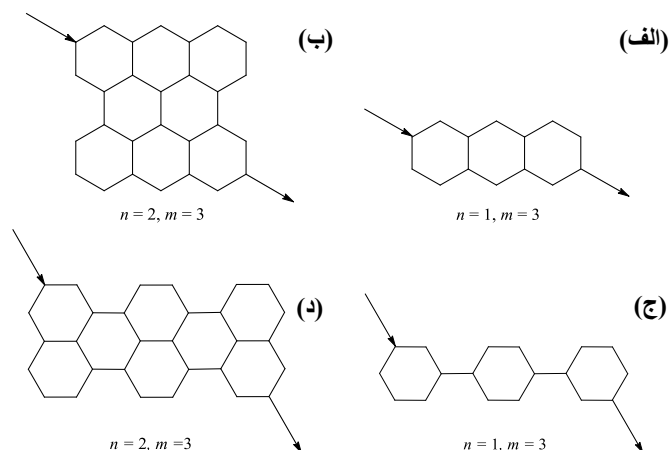
شکل ۱. چند مورد از نانونوارهای گرافن که از یک جایگاه در سمت چپ و از جایگاه متقابل در سمت راست به دو زنجیره اتمی متصل شده‌اند. (الف) و (ب) موارد زیگزآگ و (ج) و (د) موارد دسته صندلی را نشان می‌دهند. n و m به ترتیب نشان‌دهنده طول و عرض نانونوار هستند
