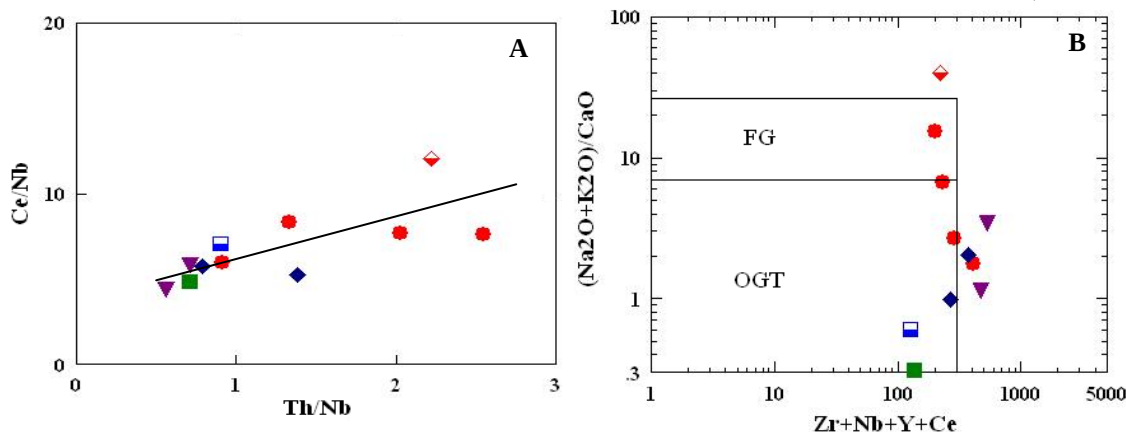
شکل ۱۱. نمودار تغییرات Ce/Nb در مقابل Th/Nb [۴۹] و (B) نمودار [۵۰]. نمادها نظیر شکل ۴ هستند
