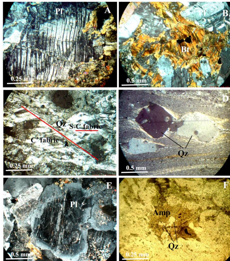
شکل ۲. A) خمیدگی ماکل‌ها در پلاژیوکلاز (Pl) مربوط به یک نمونه کوارتز دیوریتی در نور XPL، B) بلور بیوتیت (Bt) که شدیداً چین‌خورده (مجدد) است (در نور XPL). با وجود دگرشکلی شدیدی که در این‌جا اعمال شده پلاژیوکلازها (Pl) همچنان به‌صورت تیغه‌های کشیده در مقطع حضور دارند، C) بلورهای شدیداً دگرشکل یافته از کوارتز (Qz) همراه فابریک‌های S-C و C' در این تصویر مشخص شده‌اند (در نور XPL)، D) بافت چشمی در بلورهای کوارتز (Qz) در نمونه مربوط به گرانیتوئید میلوئیتی درویشان (در نور XPL)، E) پلاژیوکلاز با منطقه‌بندی نوسانی و حاشیه‌های خورده شده در یکی از نمونه‌های آنکلاو (در نور XPL) و F) تشکیل آمفیبول (Amp) در اطراف بلورهای کوارتز (Qz) (در نور PPL)
