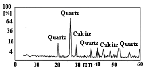
شکل ۱۱. نمونه‌ای از نمودارهای (دیفراکتوگرام‌های) XRD
