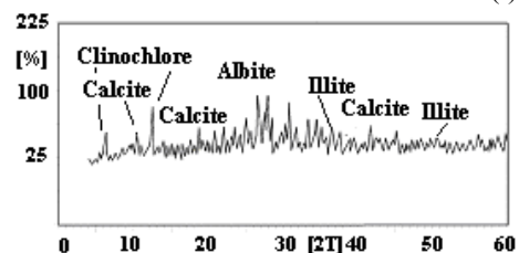
شکل ۱۱. نمونه‌ای از نمودارهای (دیفراکتوگرام‌های) XRD
