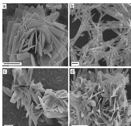
شکل ۳. تصاویر SEM فسفونات‌های فلز قلیایی خاکی (A) ساختار نانولایه‌های \text{Mg-PhPO} (b) نانوکمپندهای \text{Ca-PhPO} (c) نانولایه‌های \text{Sr-PhPO} (d) نانولایه‌های \text{Ba-PhPO}
