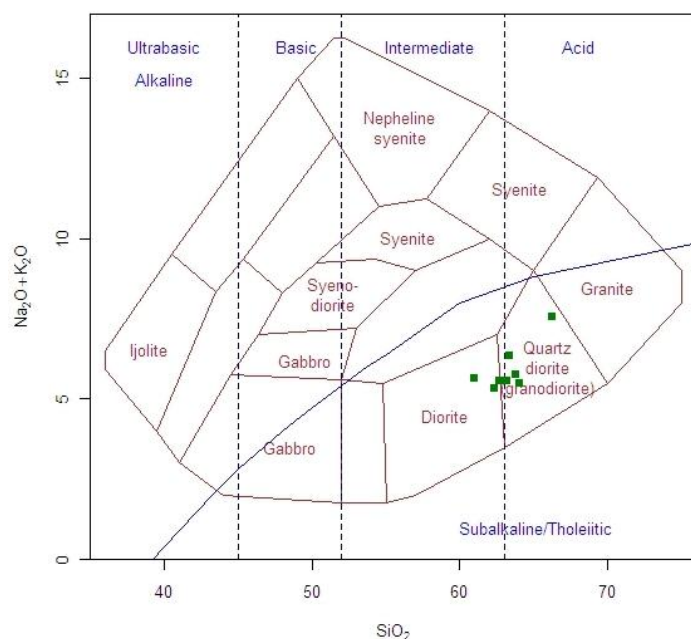
شکل ۲. موقعیت نمونه‌های بررسی شده در نمودار مجموع آلکالن (TAS) در برابر SiO ۲ [۱۷]. اغلب سنگ‌ها در محدوده ترکیبی کوچکی بین دیوریت و کوارتز دیوریت قرار گرفته‌اند
