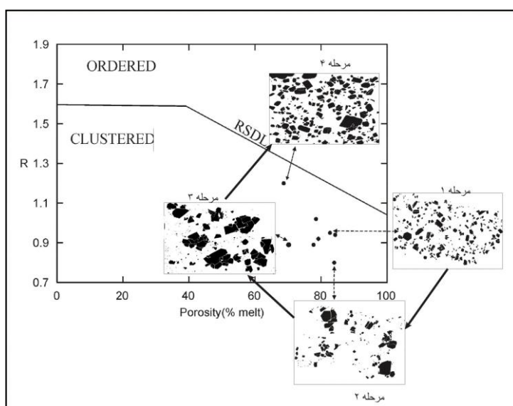
شکل ۱۰. مراحل تحول آرایش فضایی بلورها در سنگ‌های بررسی شده که بر این اساس و تلفیق با سایر اندازه‌گیری‌های بافتی، فرایندهای فیزیکی مؤثر در مخازن ماگمایی بازسازی شده‌اند. چنان‌که در این شکل دیده می‌شود، نمونه‌هایی که در مرحله ۱ تشکیل شده‌اند دارای مقدار R بزرگ‌تری هستند هر چند که در این نمونه‌ها (گروه ۱) نیز به‌دلیل هسته‌بندی ناهمگن، آرایش پلاژیوکلازها خوشه‌ای است. در ضمن اندازه بیشینه بلورها نیز کوچک‌تر از سایر مقاطع است. در مرحله ۲ به‌دلیل
