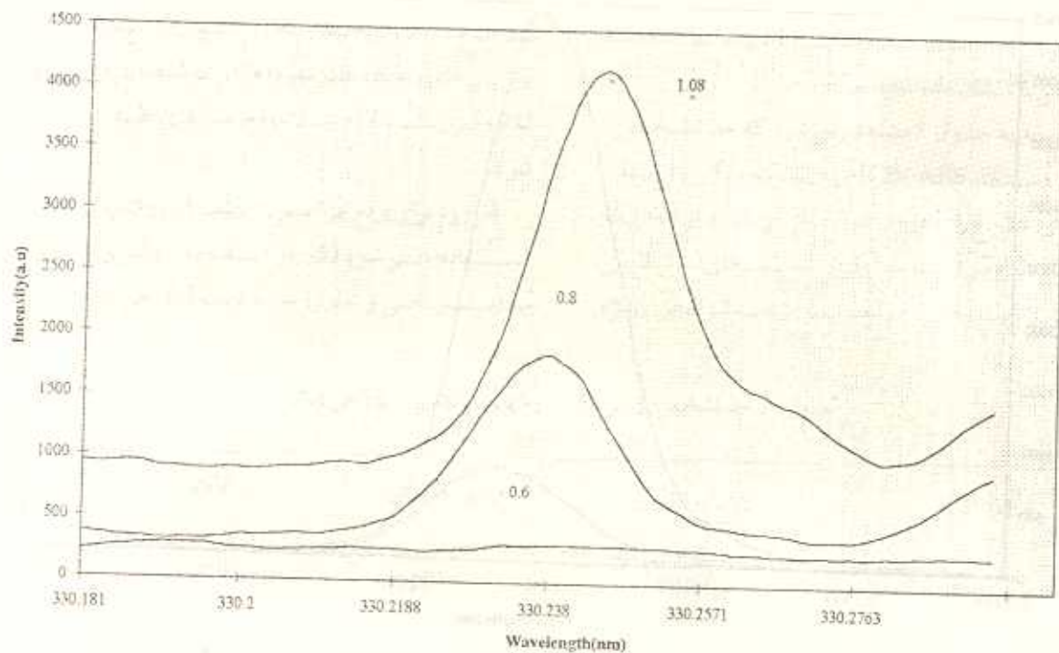
شکل ۳- اثر تغییرات توان پلاسما بر حسب کیلووات بر روی شدت نشر محلول ۳۰۰ ppmNa + ۱۰ ppmZn
