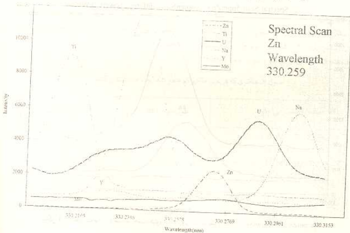
۴-۱۰۰ ppmZn + ۳۰۰ ppmNa در طول موج ۳۳۰۲۵۹ نانومتر عنصر Zn
