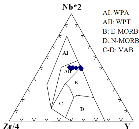
شکل ۹. موقعیت سنگ‌های منطقه جهق بر روی نمودار Nb/Zr-Y [۱۰]. محدوده‌ها به این شرح است: AI : آلکالی بازالت درون صفحه‌ای، AII : آلکالی بازالت و تولیت‌های درون صفحه‌ای، B : مورب نوع E ، D : مورب نوع N ، C-D : تولیت‌های داخل صفحه‌ای و بازالت‌های قوس آتشفشانی
