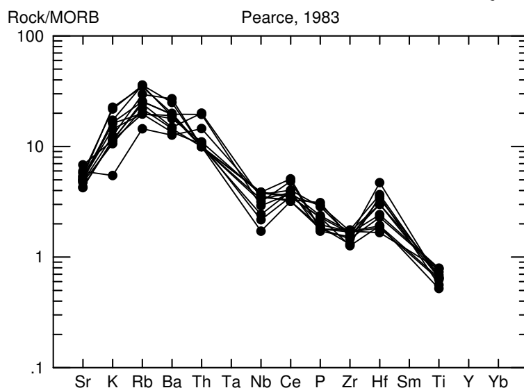
شکل ۷. الگوی فراوانی عناصر ناسازگار بازالت‌های جواهردشت به‌همچار شده با مقادیر مورب [۵]
