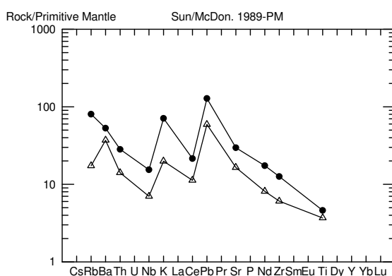
شکل ۹. مقایسه الگوی میانگین عناصر ناسازگار بازالت‌های جواهر دشت با مقادیر پوسته زیرین [۱۵] ● بازالت‌های جواهر دشت △ پوسته زیرین
