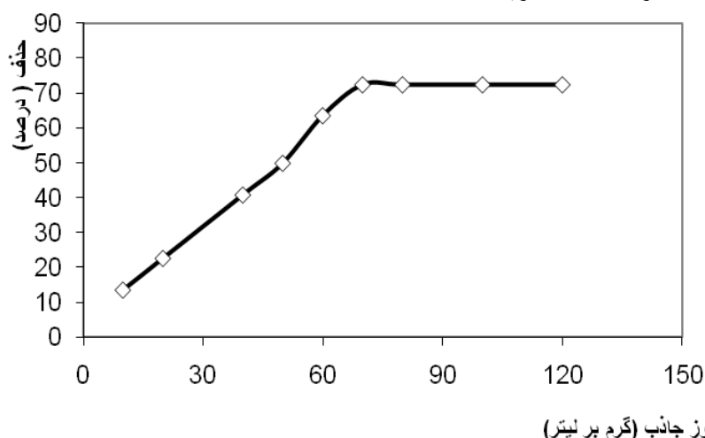
شکل ۱. منحنی درصد حذف فرمیک اسید بر حسب دوز جاذب (غلظت اولیه جذب شونده: ۰/۱ M، دما: ۲۹۵ K، مقدار جاذب: ۶g-۵/۰)
