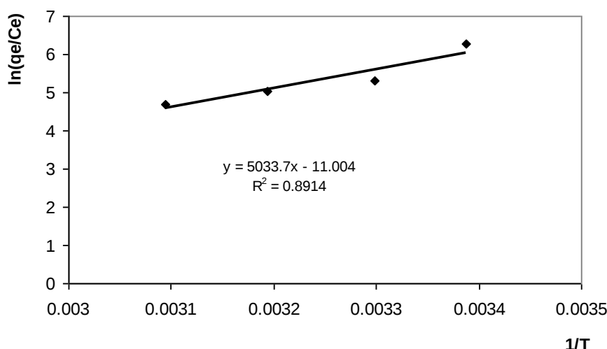
شکل ۵. منحنی تغییرات \ln \left( \frac{q_e}{C_e} \right) بر حسب 1/T برای به‌دست آوردن پارامترهای ترمودینامیکی (غلظت اولیه جذب‌شونده: ۰/۱ M، دما: ۲۹۵-۳۲۳ K، مقدار جاذب: ۳/۵ g) جدول ۲. پارامترهای ترمودینامیکی جذب فرمیک اسید روی کربن رنگبر
