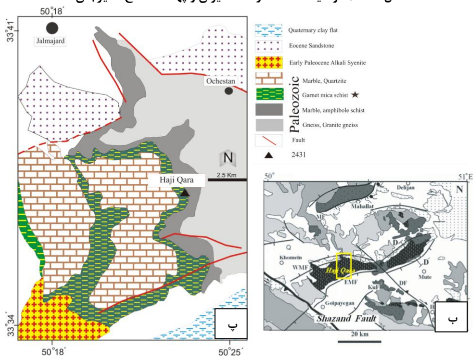
شکل ۱. ب) موقعیت گسل‌های منطقه بر روی نقشه زمین‌شناسی ۱:۲۵۰۰۰۰ گلپایگان [۳] که DF گسل دهق، EMF گسل شرق موته، WMF گسل غرب موته است (برگرفته از [۴])، پ ( نقشه زمین‌شناسی ساده شده منطقه برگرفته از نقشه زمین‌شناسی ۱:۱۰۰۰۰۰ محلات [۵] محدوده تصویر پ با مستطیل زردرنگ در تصویر ب مشخص شده است
