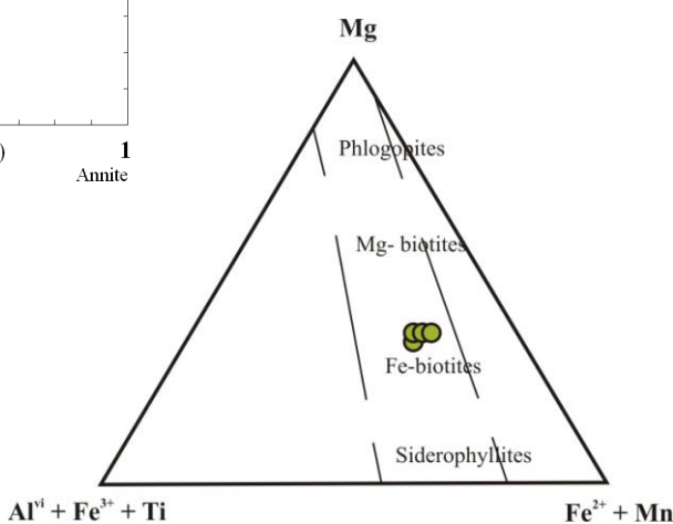
شکل ۵. قرارگیری نمونه‌های میکای سیاه در محدوده بیوتیت آهن‌دار [۱۶] (داده‌ها از جدول ۱)
