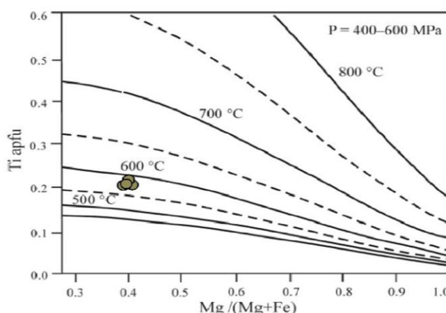
شکل ۸. منحنی‌های هم‌دما بر اساس دماسنجی تیتانیوم بیوتیت‌های مورد مطالعه [۲۵] (داده‌ها از جدول ۱)
