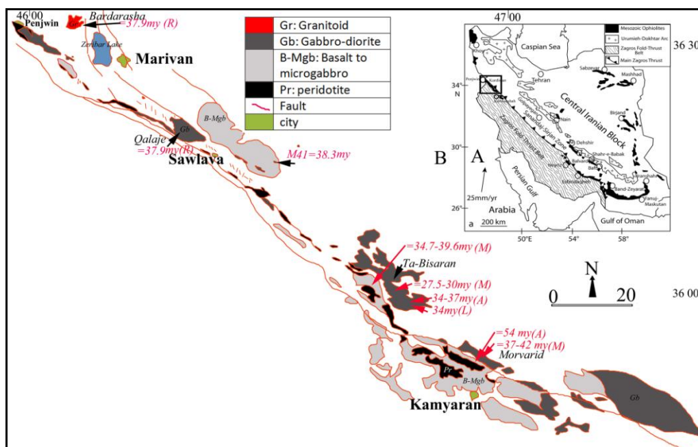
شکل ۱۲. نقشه زونبندی افیولیت‌های ایران [۳۲]، (B) نقشه پراکندگی افیولیت‌های کردستان و توده‌های گابروی و بازالتی تعیین سن شده در این پژوهش و بررسی‌های قبلی: راهنمایی سن‌های پژوهش‌های قبلی: [۱۶]، (A)، [۱۵]، (R)، [۱۱]، (M)، [۳۵]، (L).
