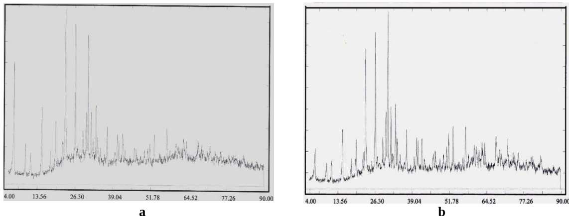
شکل ۴. الگوهای XRD (a) X_{13} و (b) Nano-MnO_2/Zeolite\ 13X
