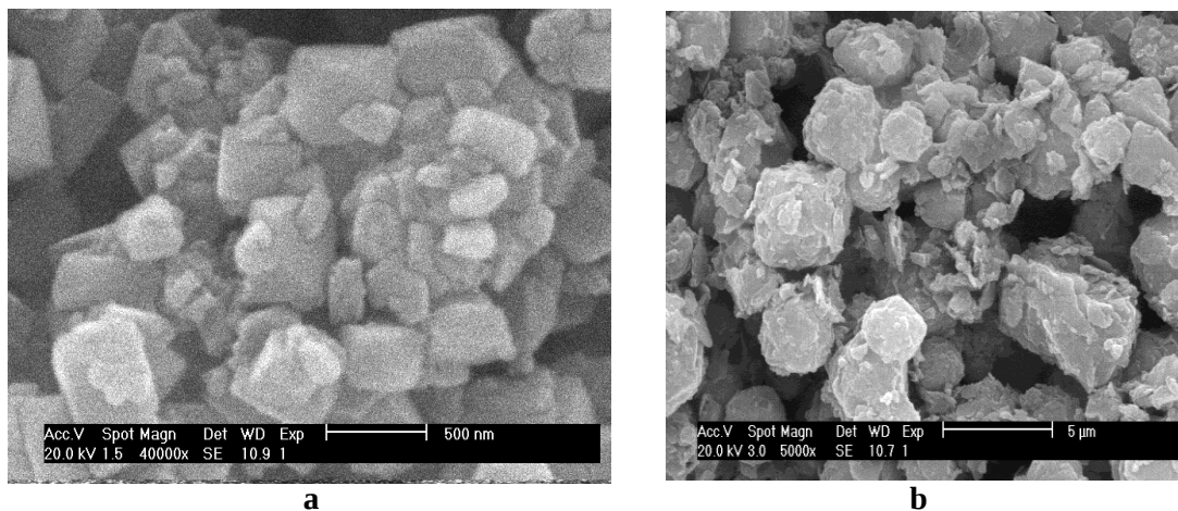
شکل ۵. الگوهای SEM (a) X_{13} و (b) Nano-MnO_2/Zeolite\ 13X
