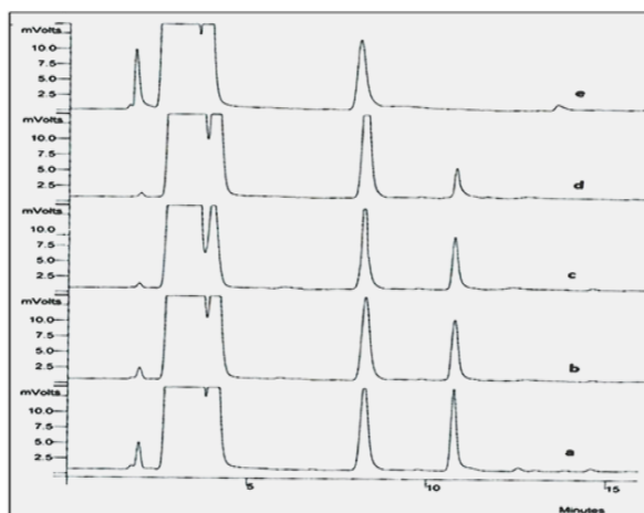
شکل ۸. کروماتوگرام GC واکنش نانوکامپوزیت یا شبه عامل CEES-۲ در حلال هپتان
