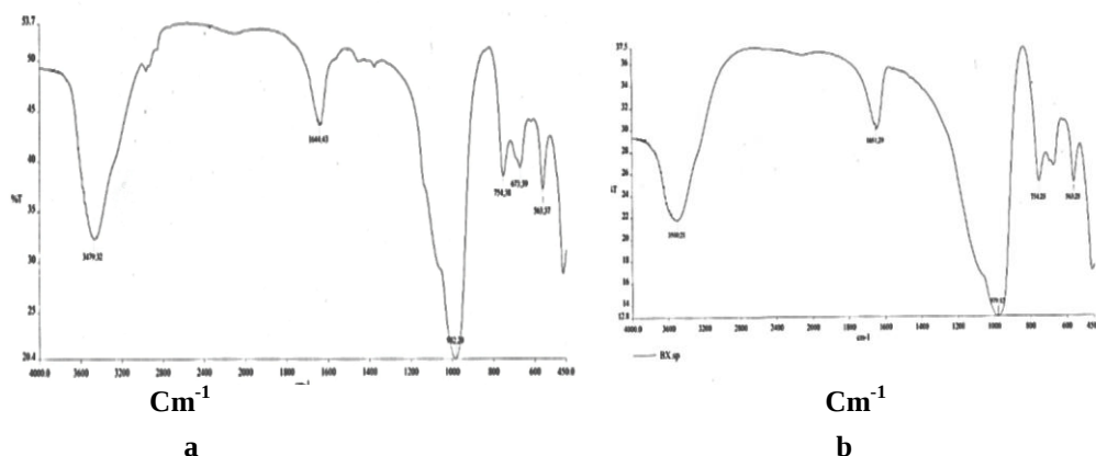
شکل ۶. طیف‌های FT IR (a) ۱۳X و (b) Nano-MnO 2 /Zeolite 13X
