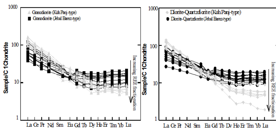
شکل ۷. مقایسه الگوی تغییرات فراوانی عناصر خاکی نادر در توده‌های نفوذی تیپ جبال بارز و تیپ کوه پنج که نسبت به کندریت C1 به‌هنجار شده‌اند. غنی‌شدگی کمتر گرانیتویدهای کوه پنج از عناصر خاکی نادر متوسط و سنگین نسبت به گرانیتویدهای جبال بارز به‌وضوح با قرار گرفتن روندهای مربوط به عناصر مذکور در آن‌ها در زیر روندهای مربوط به گرانیتویدهای جبال بارز آشکار است
