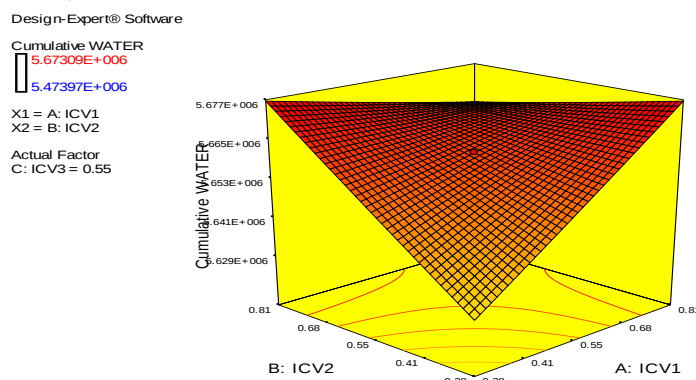
شکل ۹. (b) نمودار مدل آب تجمعی برای ICV1 و ICV2 به روش RSM (دوره زمانی اول)
