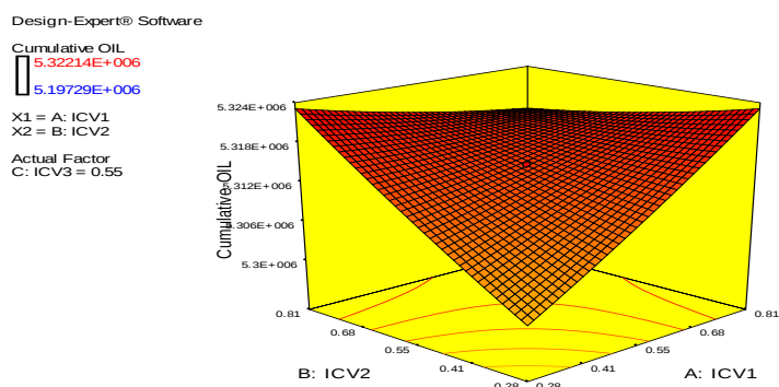
شکل ۹. (a) نمودار مدل نفت تجمعی برای ICV1 و ICV2 به روش RSM (دوره زمانی اول)
