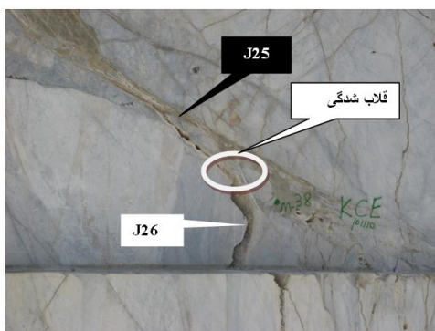
شکل ۱۷. نمایی از دو درز J25 و J26 و ساختار قلاب‌شدگی (دید به سمت شمال خاور)
