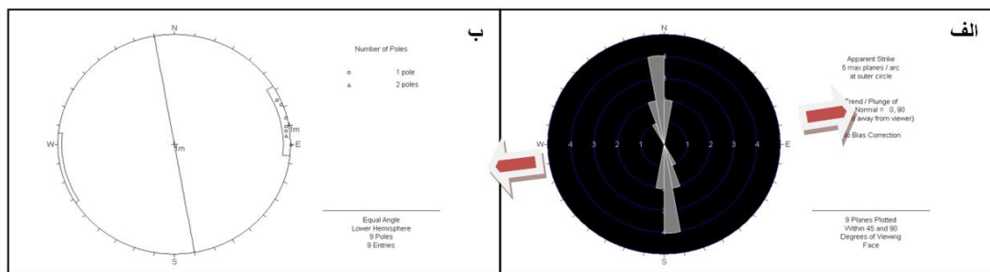
شکل ۲۰. الف) تصویر صفحه‌ی میانگین امتداد دسته درزه‌های با شیب ۹۰ درجه در نرم افزار DIPS 5.1
