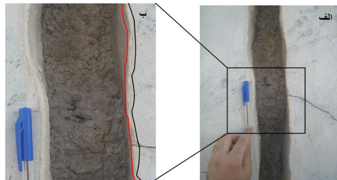
شکل ۱۱. الف و ب) تصاویر درز J19، دو نسل پرشدگی قدیمی کلسیت S1 و S2 در حاشیه دیواره درز مشخص شده است، درزه از محل پرشدگی S2 باز شده و در حال پرشدن با رس است
