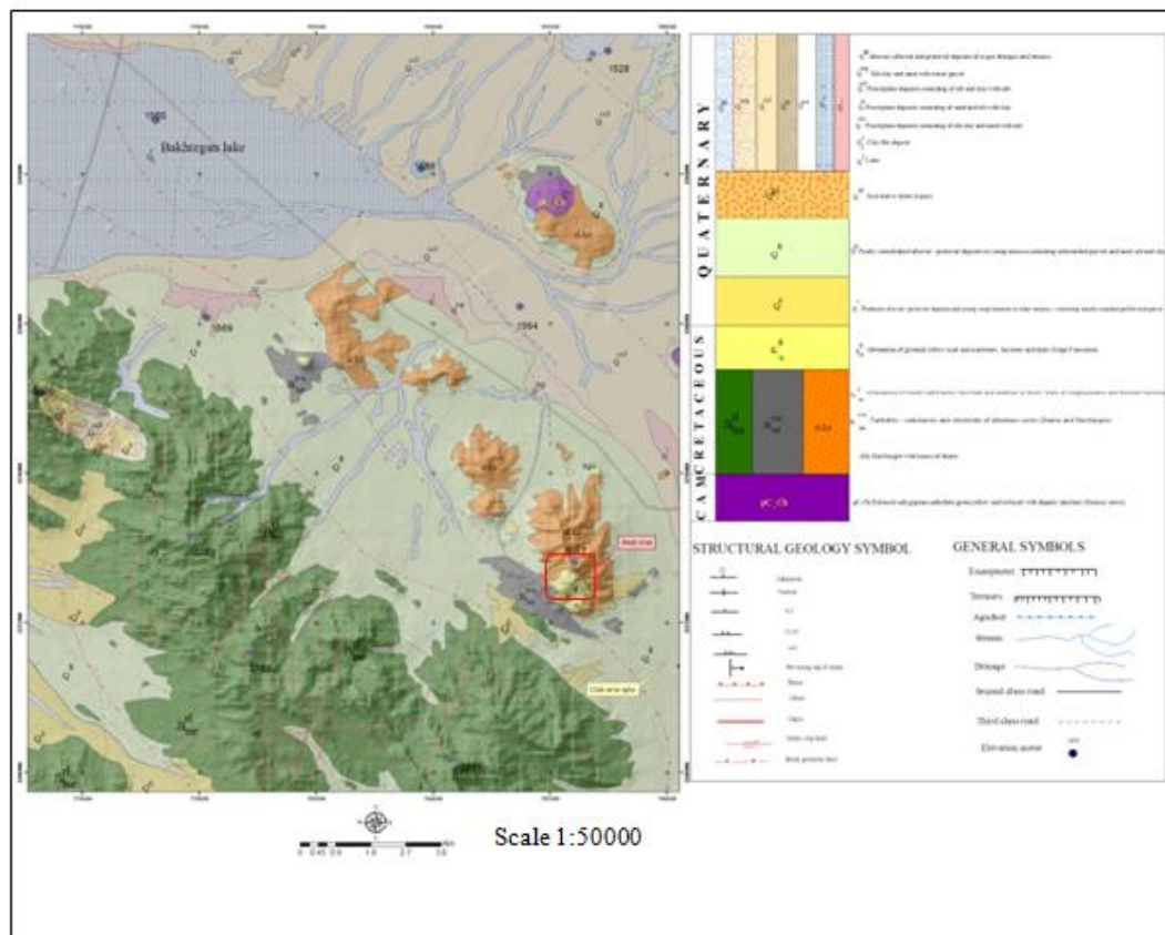
شکل ۳. نقشه زمین‌شناسی منطقه جنوب خاور آغاده- طشک منطقه داخل محدوده قرمز منطقه بررسی شده است
