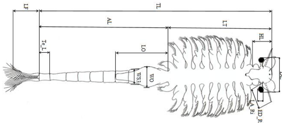
شکل ۲. صفات ریختی: طول کل بدن (TL)، طول شکمی (AL)، طول سینه (LT)، طول سر (HL)، طول فورکا (LF)، طول تلسون (TL)، قطر چشم راست (ED-RI)، طول شاخک راست (LA-RI)، فاصله بین دو چشم (DE)، عرض بند سوم شکمی (WS3)، طول رحم (LO)، عرض رحم (WO).
