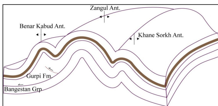
شکل ۴. بلوک دیاگرامی از تاق‌دیس‌های فرعی در پهلوه‌های تاق‌دیس زنگول
