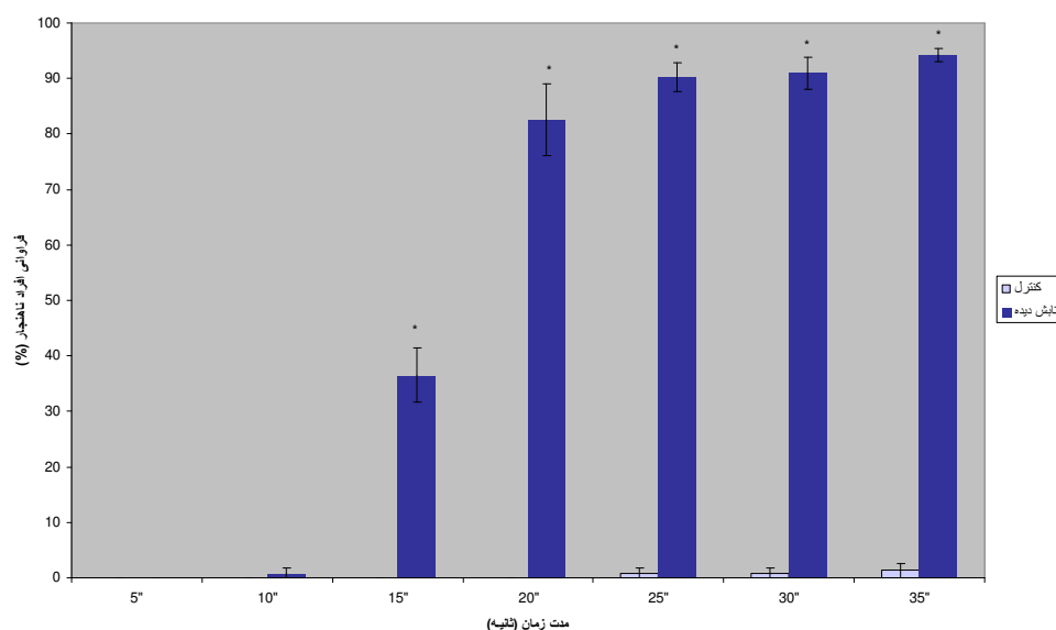
شکل ۵. نمودار اثر مدت زمان تابش بر درصد فراوانی افراد دارای ناهنجاری در گروه اشعه دیده با UV و گروه کنترل ( P < 0.01 )
