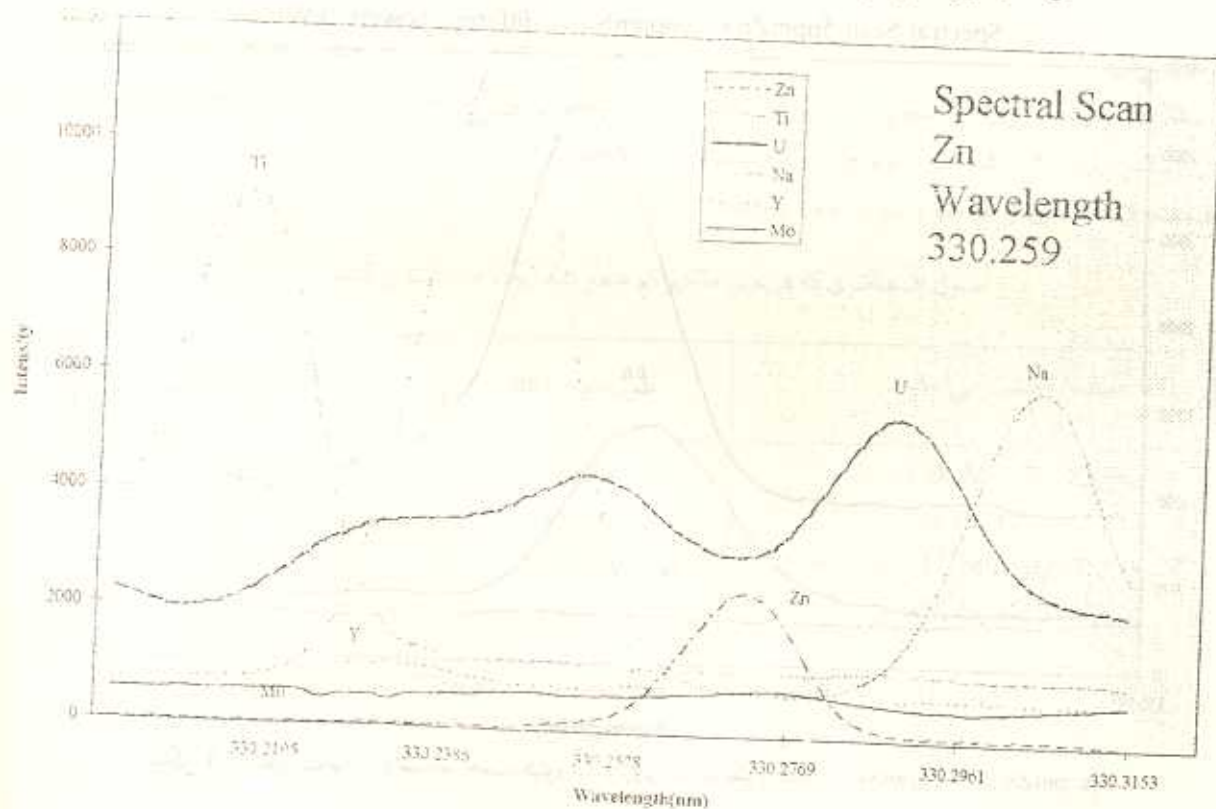
۴- طیف نشری عناصر Ti, U, Na, Y, Mo در طول موج ۳۳۰۲۵۹ نانومتر عنصر Zn
