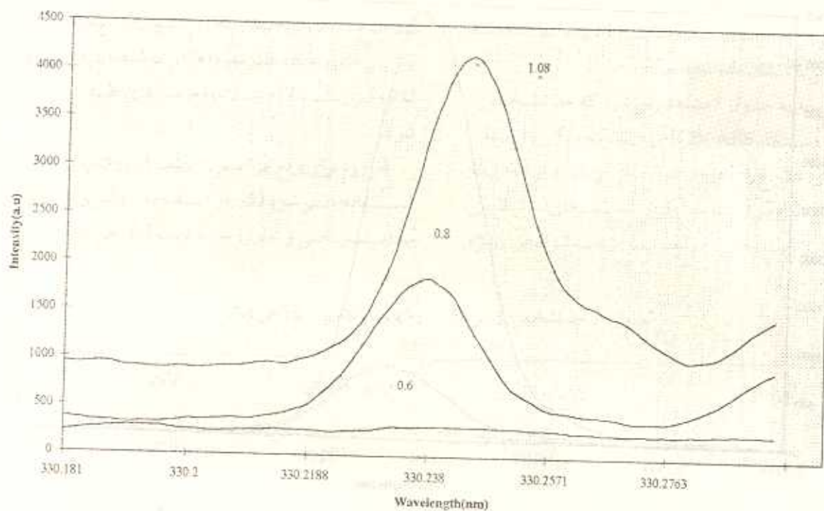
شکل ۳- اثر تغییرات توان پلاسما بر حسب کیلووات بر روی شدت نشر محلول ۳۰۰ ppmNa + ۵۰ ppmZn
