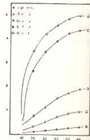
شکل ۸- تاثیر محلول HCl + اتیلن گلیکول روی حذف آهن
