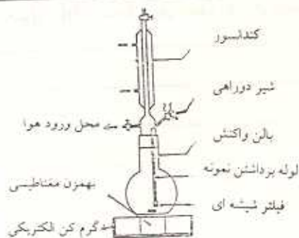
شکل ۱- شمای دستگاه کانی شونی ایلمنیت
