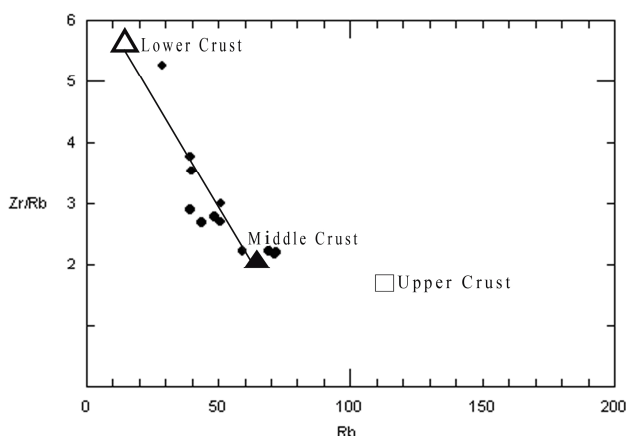
شکل ۱۷. نمودار نیمه لگاریتمی تغییرات Zr/Rb در برابر Rb از آسکرن و همکاران [۲۷]. مقادیر میانگین پوسته زیرین و میانی از رودنیک و فونتین [۱۵] و پوسته بالایی از تیلور و مک لان [۱۹] اقتباس شده است
