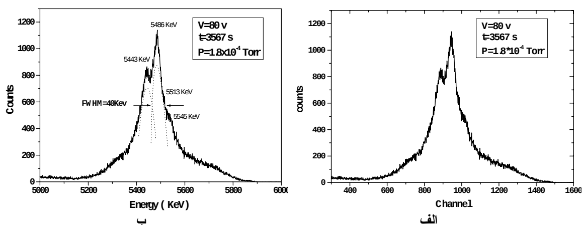
شکل ۲. الف) طیف ذرات آلفای 5/48\text{ MeV} از چشمه ^{241}\text{Am} آشکار شده با آشکارساز \text{GaAs} با تماس شاتکی دایره‌ای شکل به قطر 3\text{ mm} و ضخامت 400\text{ }\mu\text{m} ، ب) طیف انرژی ذرات آشکار شده شکل ۲. الف
