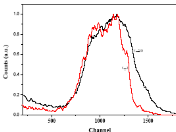
شکل ۵. طیف آلفای اندازه‌گیری شده MeV\ 0.48 از چشمه ^{241}Am آشکار شده با آشکارساز GaAs با تماس شاتکی دایره‌ای شکل به قطر 2\text{ mm} و ضخامت 400\text{ }\mu\text{m} در ولتاژهای مختلف
