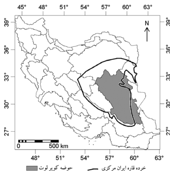
شکل ۱. محدوده پهنه رسوبی - ساختاری خارده قاره ایران مرکزی و موقعیت حوضه هیدرولوژیکی کویر لوت (بر اساس تقسیم‌بندی آقا نباتی، ۱۳۸۳)
