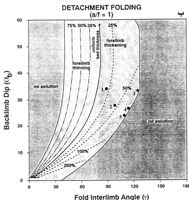
شکل ۶- الف) داده‌های لازم جهت تحلیل نازک شدگی و یا ضخیم شدگی یال جلویی چین‌های جدایشی، ب) نمودار نازک شدگی و ضخیم شدگی یال جلویی چین‌های جدایشی مورد اشاره در جدول بالا، اقتباس از [۹]
