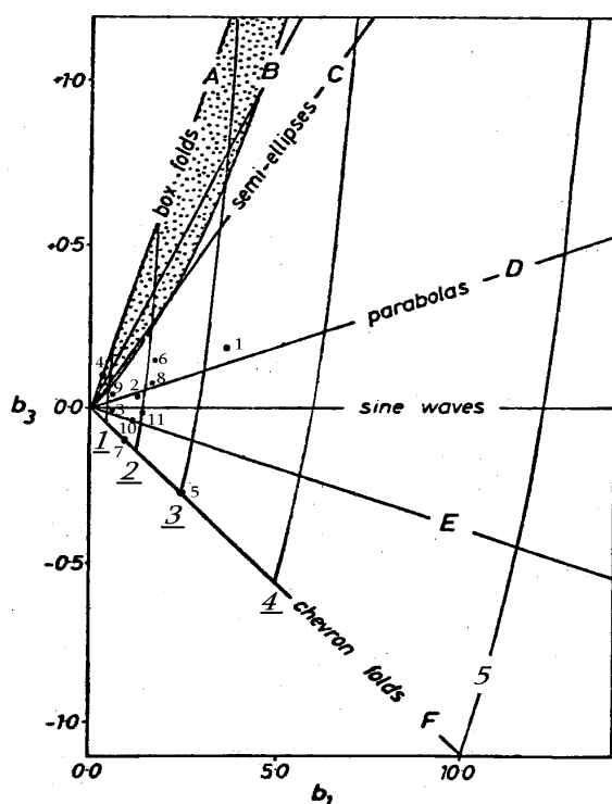
شکل ۳- روش ترسیمی برای رسم شکل چین‌ها، اقتباس از [۴]. خطوط ۱ تا ۵ مربوط به دامنه چین و نقاط، نشان‌گر چین‌های ذیل هستند:
