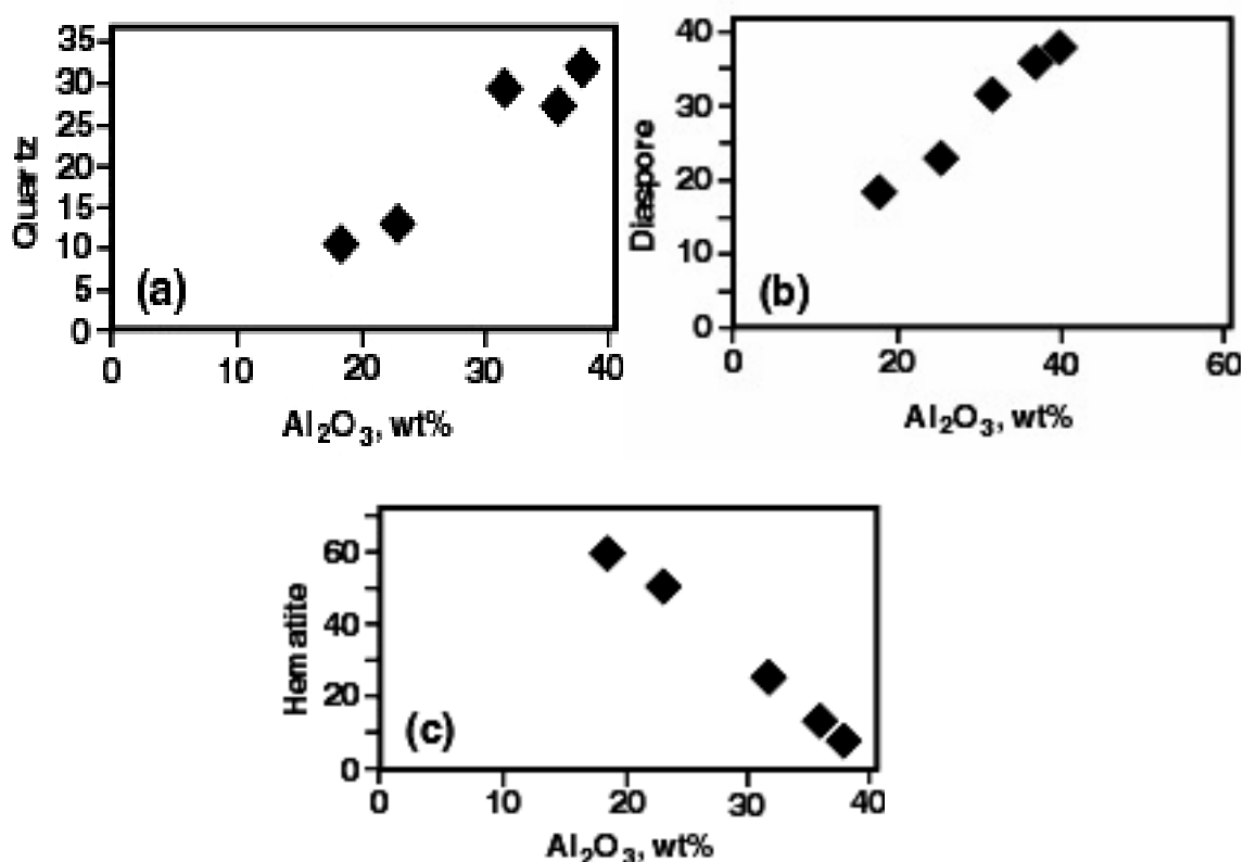
شکل ۳- تغییرات کانی‌های کوارتز، هماتیت و دیاسپور در مقابل تغییرات مقادیر درصد وزنی \text{Al}_2\text{O}_3 کل در واحدهای بوکسیتی قبی
