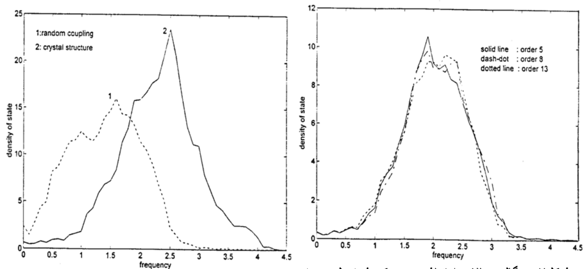
شکل ۷- چگالی حالات ارتعاشی در یک شبه بلور سه بعدی 25 \times 25 \times 25 اتمی در سه حالت با تناوب‌های فیبوناچی ۵، ۸ و ۱۳. (بارزتر شدن شبه گاف با افزایش تناوب فیبوناچی قابل توجه است)
