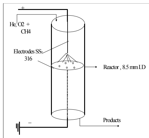
شکل ۲- رآکتور کرومائی مثبت
