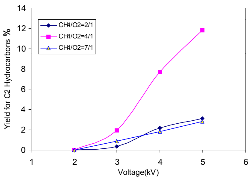
شکل ۶ الف- تاثیر ولتاژ در راندمان نهادهی به هیدروکربن‌های \text{C}_2 در سطوح مختلف نسبت خوراک در دمای ۶۵۰ درجه سانتی‌گراد
