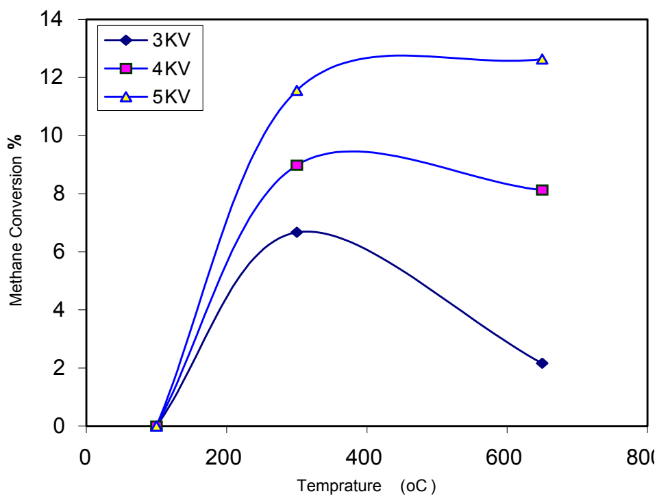
شکل ۱۰ الف- تاثیر دما در تبدیل متان در نسبت خوراک \text{CH}_4/\text{O}_2=4/1
