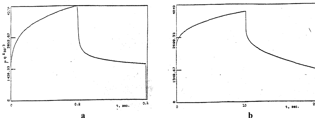
شکل ۴- (a) منحنی کروئوکولومتری الکترود نازک طلا 300 \text{ \AA} در الکترولیت 0.1 \text{ M LiClO}_4
