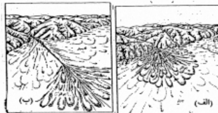
شکل ۱-الف- تشکیل مخروط افکنه در مجاور پیشانی گسلی فعال (ب) تشکیل مخروط افکنه در پیشانی غیرفعال (Keller, 1986)
