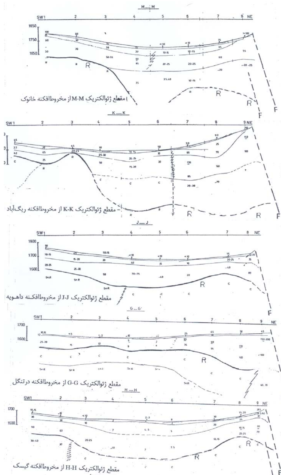
شکل ۹- مقاطع ژئوالکتریک از مخروط افکنه‌های دشت زرنده
