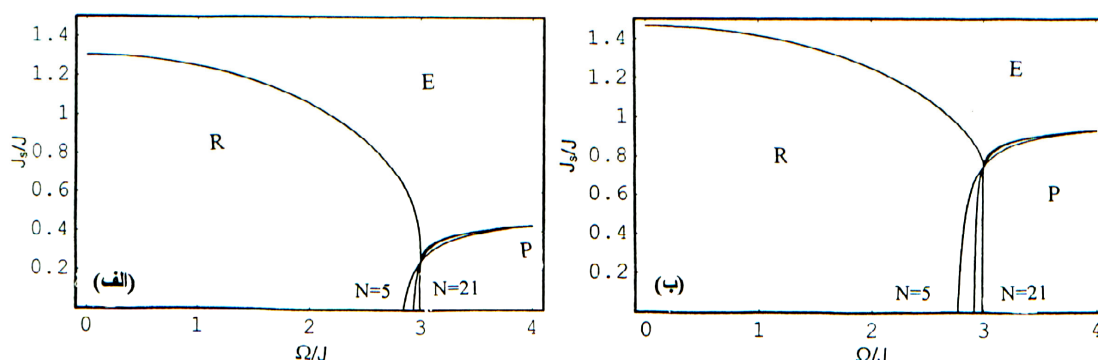
شکل ۲. دیاگرام‌های فاز در صفحه (\Omega_s/J, J_s/J) برای فیلم‌هایی با یک لایه سطحی ( N_s=1 ) که در آن مربوط به فاز کاهش یافته (T_c(\text{film}) < T_c(\text{bulk})) و مربوط به فاز افزایش یافته (T_c(\text{film}) > T_c(\text{bulk})) و فاز P پارالکترونیک است. (الف) \Omega_s/J=1 (ب) \Omega_s/J=2
