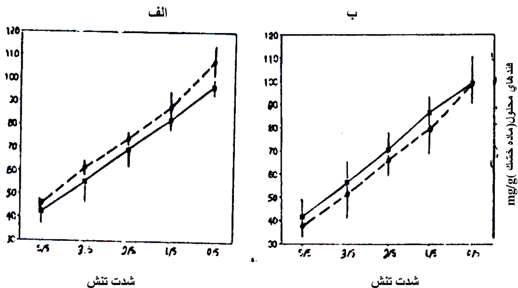
شکل ۲. مقایسه اثر تنش آبی بر تغییرات قندهای محلول الف) در ساقه دو رقم کاکا و (---) و جم و ب (■■■) در ریشه نخود
