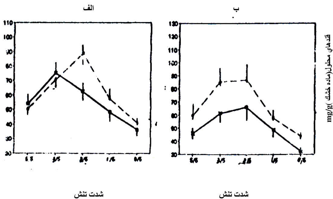
شکل ۲. مقایسه اثر تنش آبی بر تغییرات قندهای محلول الف) در ساقه دو رقم کاکا و (---) و جم و ب (■■■) در ریشه نخود
