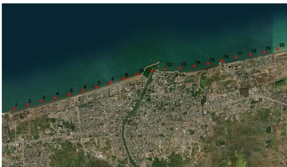
شکل ۷. الگوی تغییرات مکانی خط ساحل محدوده شهر بابلسر در سال ۱۳۷۴ نسبت به سال ۱۳۵۶؛ موقعیت اندازه‌گیری تغییرات با شناسه نقاط مشخص است که متناظر با آن را می‌توان با نقاط نمایش داده شده بر روی تصویر ماهواره‌ای می‌توان مشاهده نمود.
