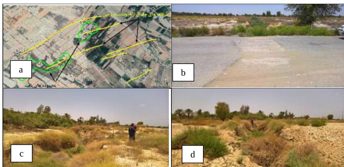
شکل ۱۰: a: موقعیت شکاف های ناشی از فرونشست زمین در اطراف روستای دول آباد، b، c و d: شکاف های ناشی از فرونشست زمین و آسیب به منازل در روستای دوآباد، e: موقعیت شکاف های ایجاد شده در روستای کهورنانجک (خطوط زرد) و محدوده های در معرض آسیب بافت مسکونی (هاشور قرمز) f، g و h: موقعیت شکاف های ناشی از فرونشست زمین در روستای کهورنانجک، i: موقعیت شکاف های ایجاد شده در محدوده پیرامونی بافت مسکونی روستای دره شور (خطوط زرد) و محدوده های در معرض آسیب بافت مسکونی (هاشور قرمز)، j: تصویری از شکاف ناشی از فرونشست زمین در روستای دره شور
