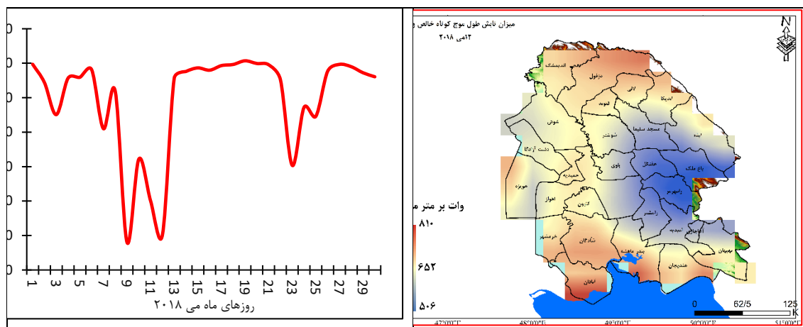
شکل ۵- توزیع زمانی (ماهانه) و مکانی داده های باز تحلیل شده ساعتی میزان تابش خالص موج کوتاه ورودی به سطح زمین (SNSR) در سطح استان خوزستان (مستخرج از پایگاه اقلیمی اروپایی ECMWF نسخه ERA۵ (در ساعت ۱۲ ظهر یا ۰۹ UTC)
