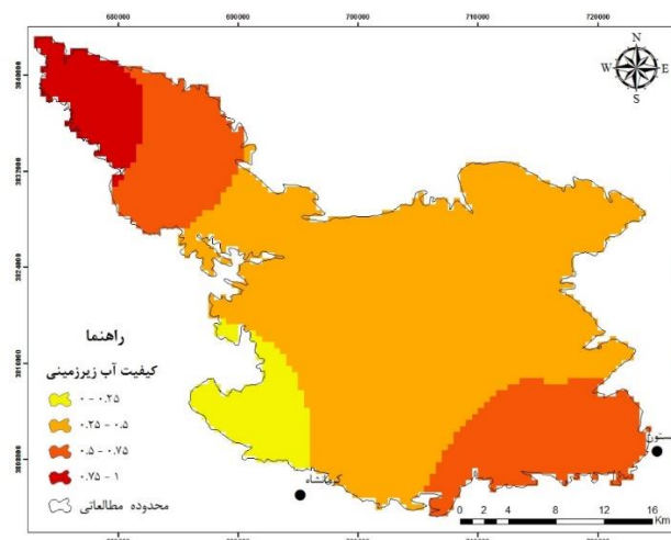
شکل (۱۰). پراکندگی آلودگی آب زیرزمینی بیستون و پراو
