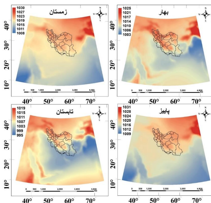
شکل ۴. الگوی فصلی فشار (بر واحد هکتوپاسکال) مشاهداتی ایران طی دوره ۱۹۶۰-۲۰۰۵ بر اساس مدل HadGEM ۲ -ES
