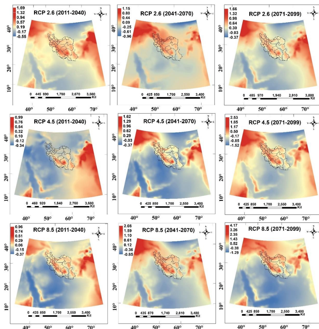
شکل ۸ - ناهنجاری فشار (بر واحد هکتوپاسکال) تراز دریا SLP فصل پاییز طی دوره آینده نزدیک (۲۰۴۰-۲۰۱۱)، آینده میانی (۲۰۷۰-۲۰۴۱) و آینده دور (۲۰۹۹-۲۰۷۱) بر اساس مدل HadGEM ۲ -ES تحت سناریوهای واداشت تابشی RCPs
