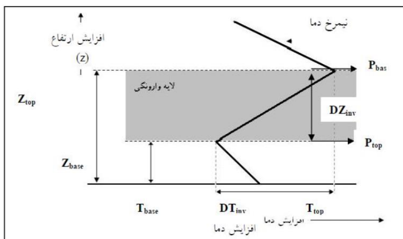
شکل (۲). خصوصیات نيمرخ وارونگی دمای هوا (یاکوبلیس و همکاران، ۲۰۰۹)
