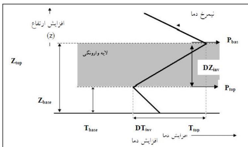
شکل (۲). خصوصیات نیمرخ وارونگی دمای هوا (باکوبلیس و همکاران، ۲۰۰۹)
