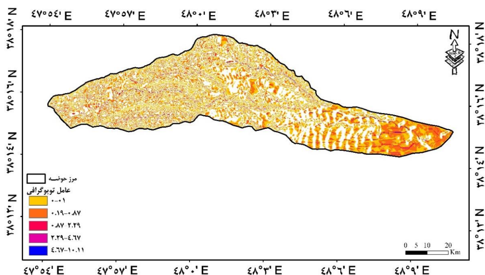
شکل ۷: شاخص توپوگرافی (LS) حوزه آبخیز عموقین.
